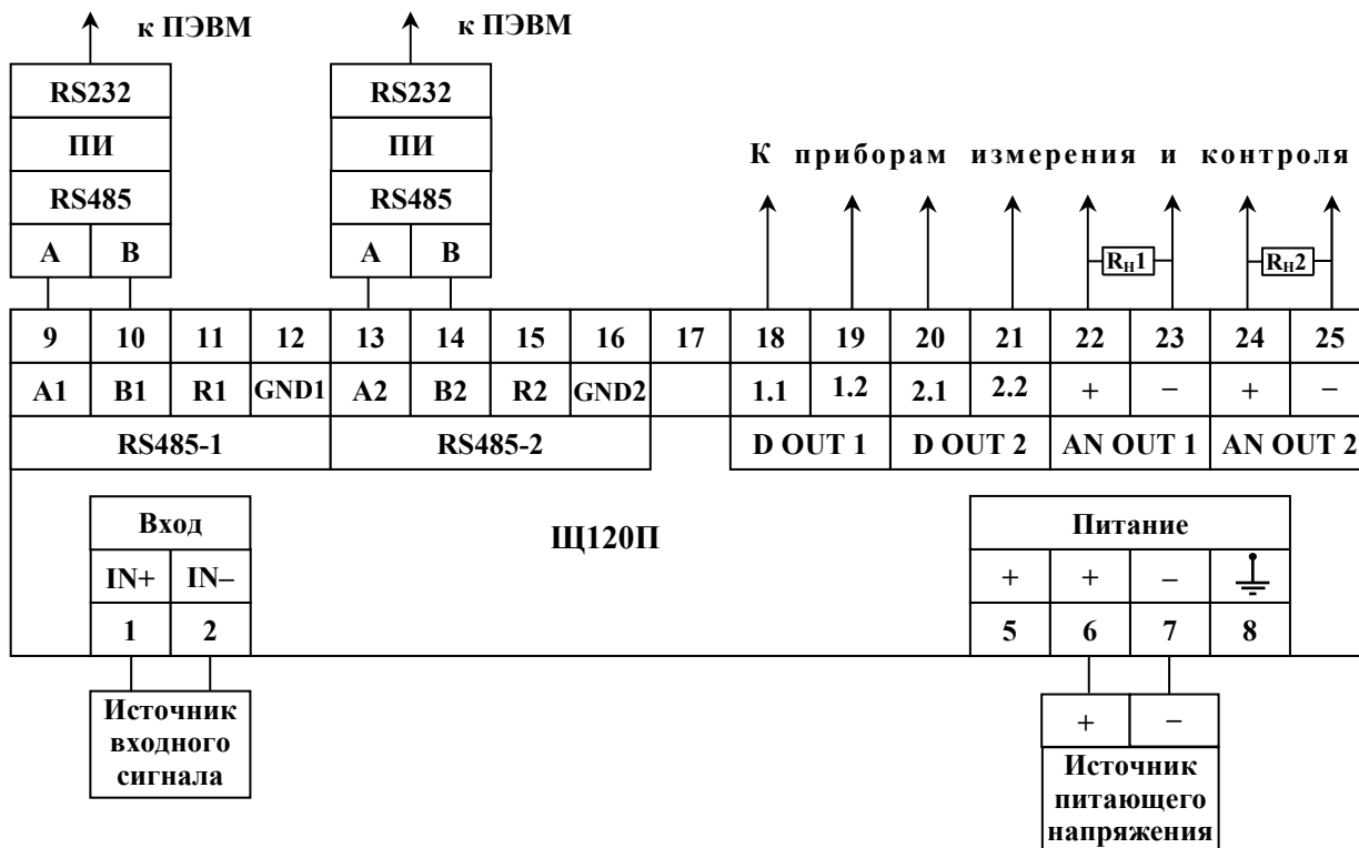
Рисунок Б.3 – Схемы подключения приборов Щ96П
